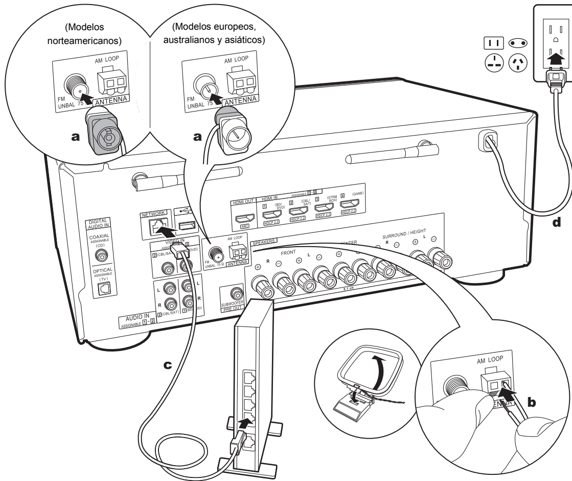
a Antena FM para interiores, b Antena AM para interiores, c Cable Ethernet, d Cable de alimentación
